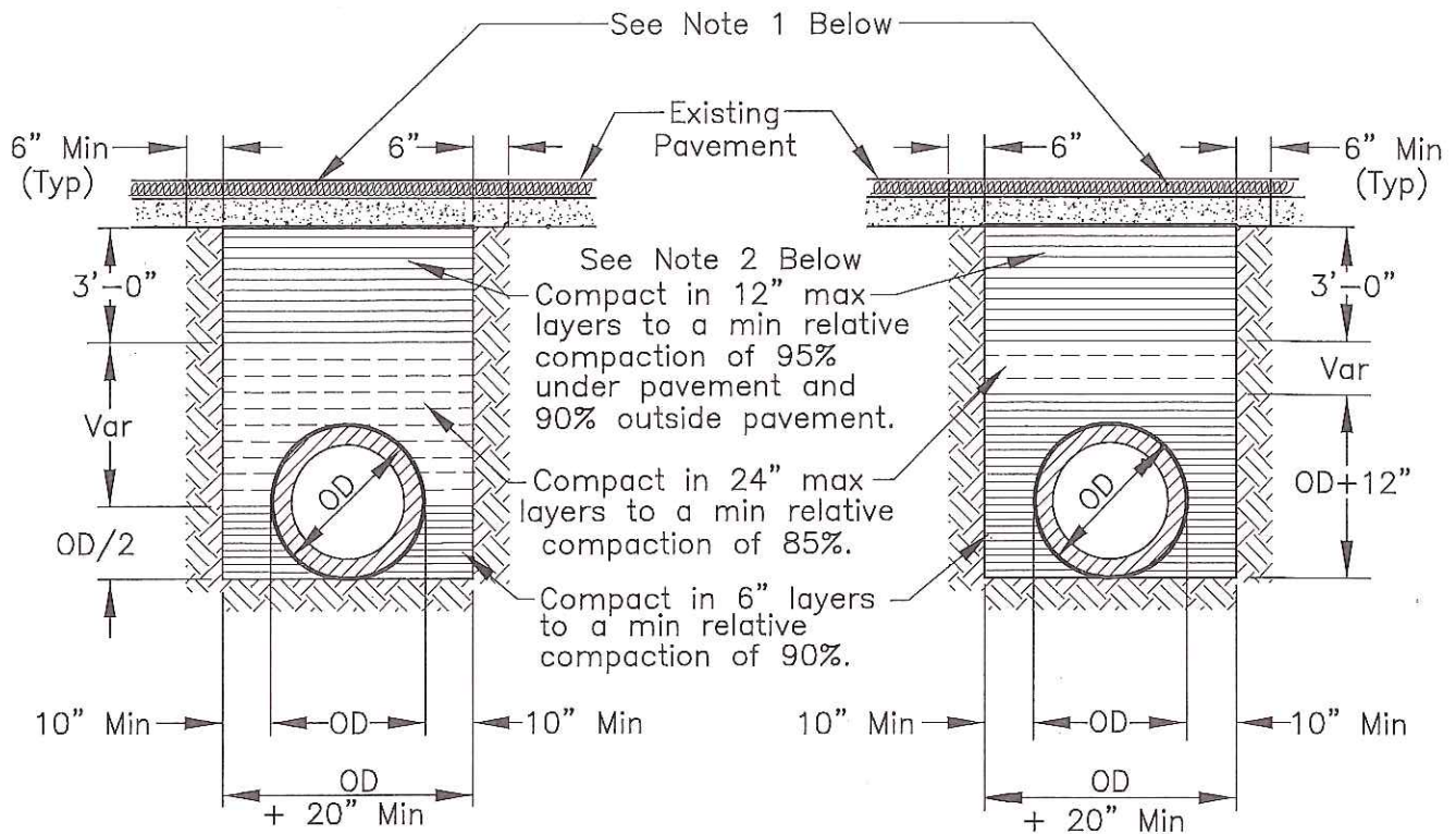
RIGID CONDUIT
